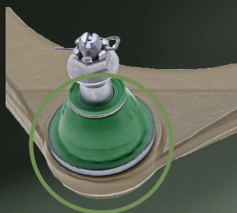
SOLUTION BREVETÉE DYNAMIC CONTROL BEARING™ Optimise la durée de vie en supportant la précharge. Les paliers frittés conservent leurs performances dans des conditions de températures et des charges élevées
