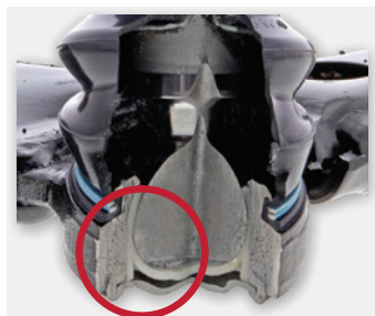
JOINT À ROTULE Roulement en plastique non graissable
