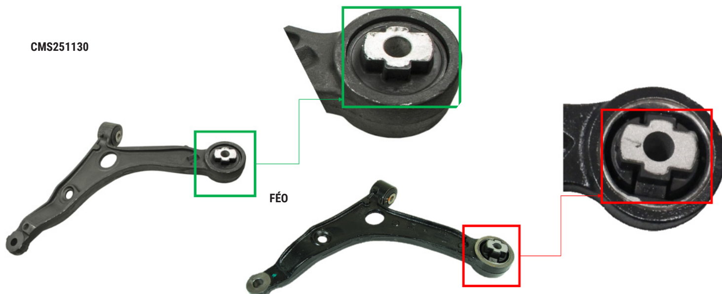
Figure 1. Bras de suspension inférieur avant Mevotech Supreme CMS251130 avec conception de bague améliorée (gauche) par rapport à la bague standard du fabricant d'équipement d'origine (droite)
